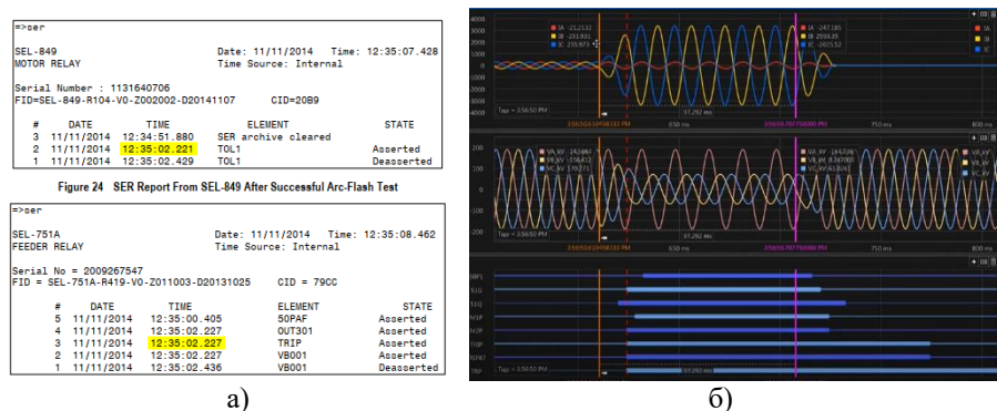
1-сурет. QuickSet бағдарламасында доғалық қорғаныстың жұмыс жасау есебі (а) мен апаттық режимді жазған осциллограммасы (б)
